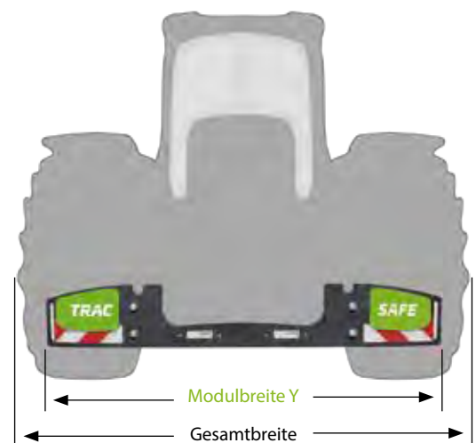
Modul-Zuordnung Gesamtschlepperbreite abzgl. 20cm = TRACSAFE Modulbreite
